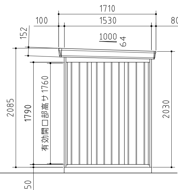
側面図
