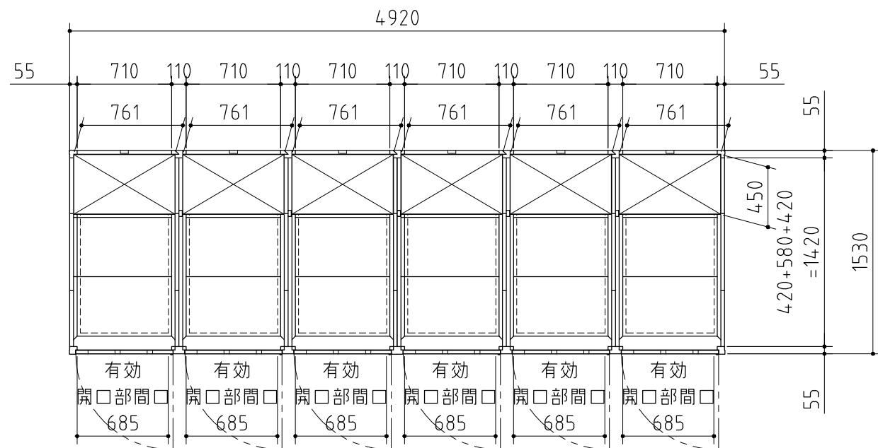
平面図
